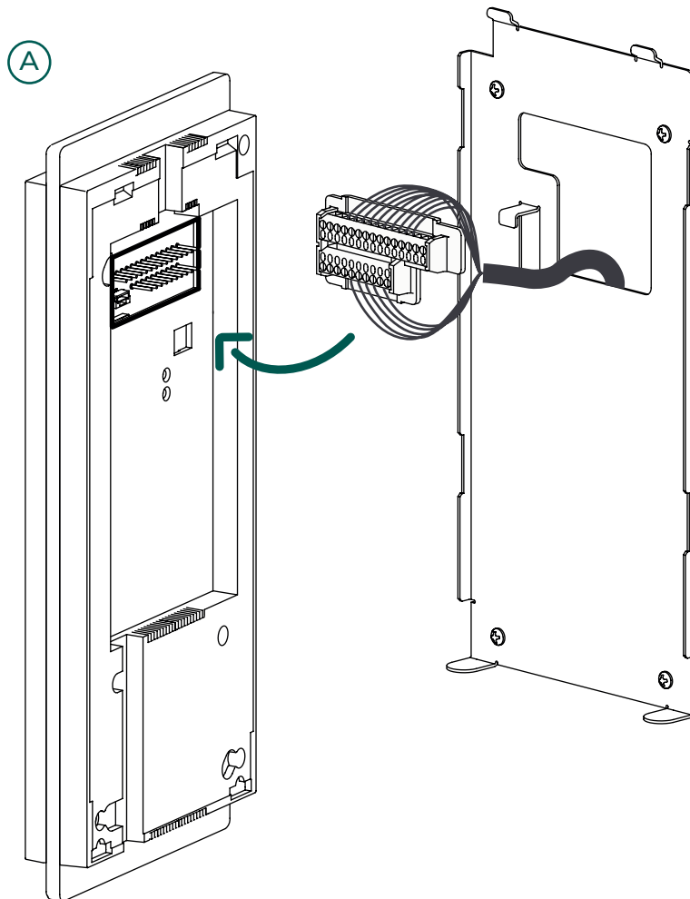
Entrada cables desde canaleta Cable entry from the cable conduit. Entrada cables des de canaleta.
